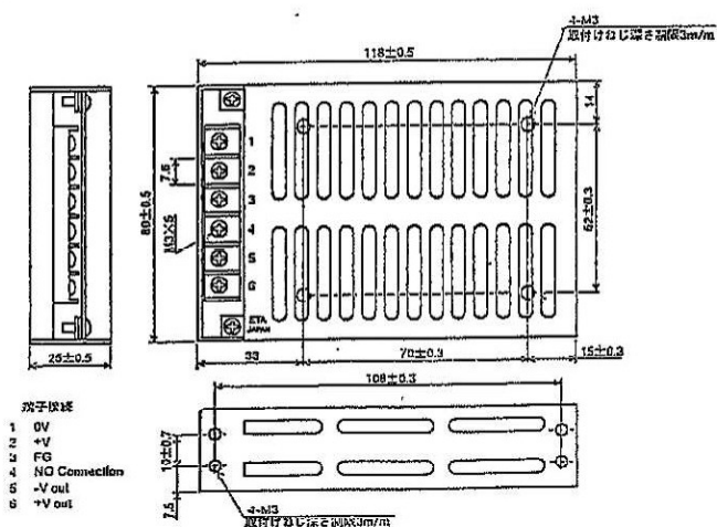
■ VTM-SC・SDシリーズ (15W) 単出力
