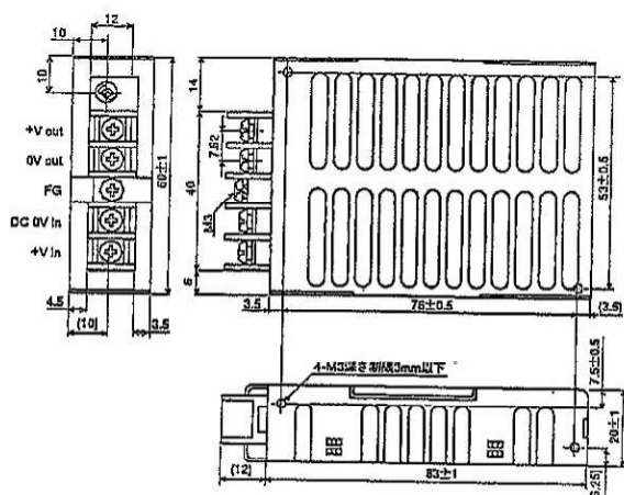
■ SVM-SC・SDシリーズ(15W) 準出力
