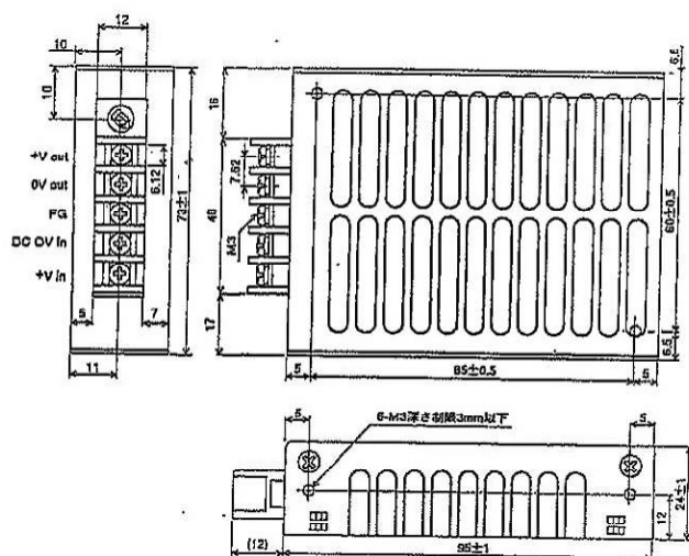
■ SVA-SC・SDシリーズ (25W) 単出力
