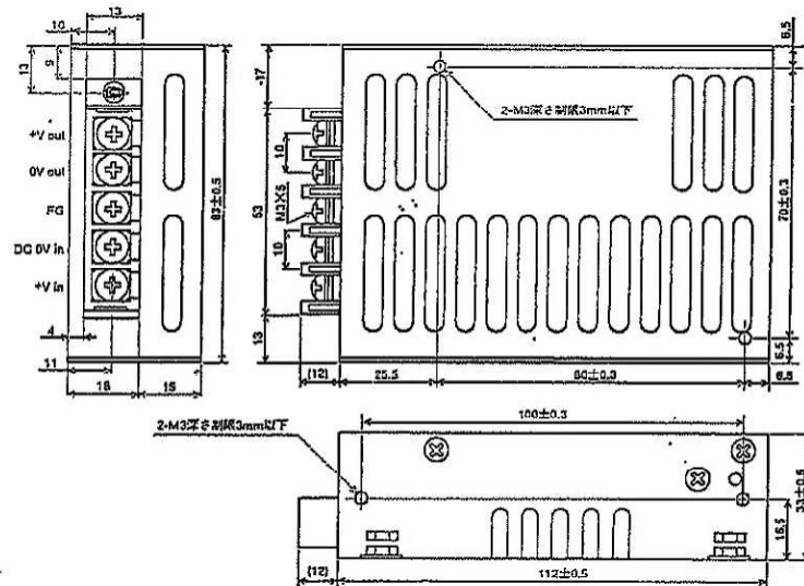
■ SVB-SC・SDシリーズ (50W) 単出力
