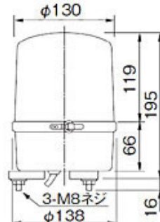
取付面寸法図
