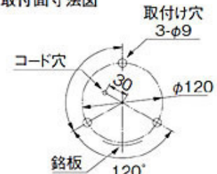
取付面寸法図
