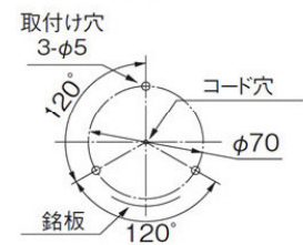
取付面寸法図
