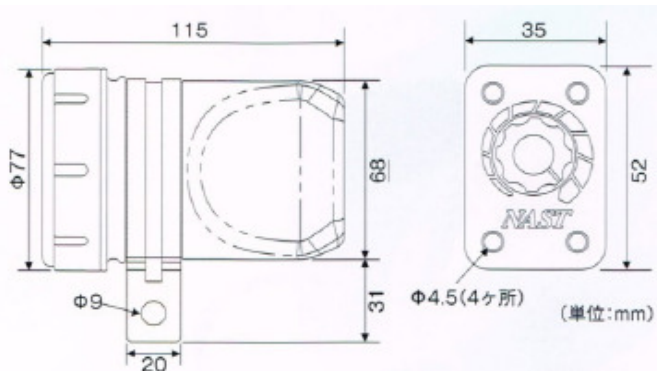
【外観寸法図】
