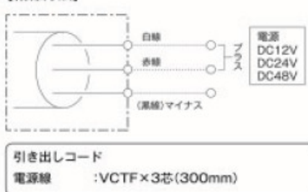
【結線方法】
