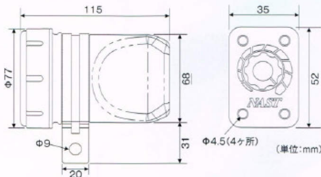
【外観寸法図】
