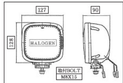
寸法図
