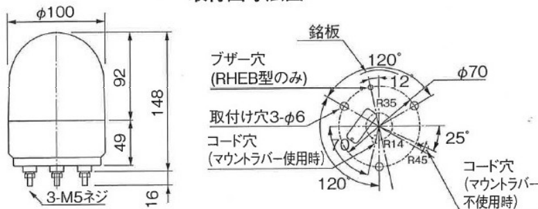
取付面寸法図
